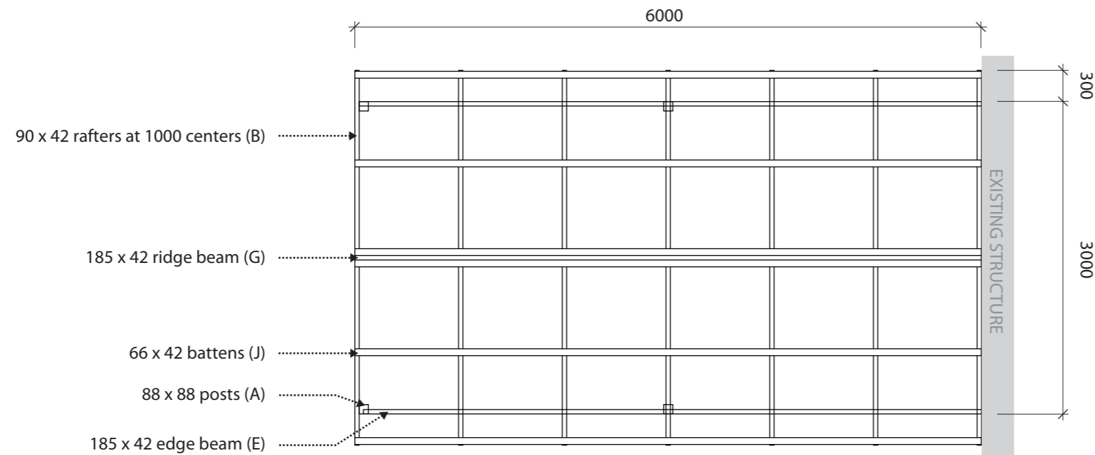
○ ROOF PLAN
